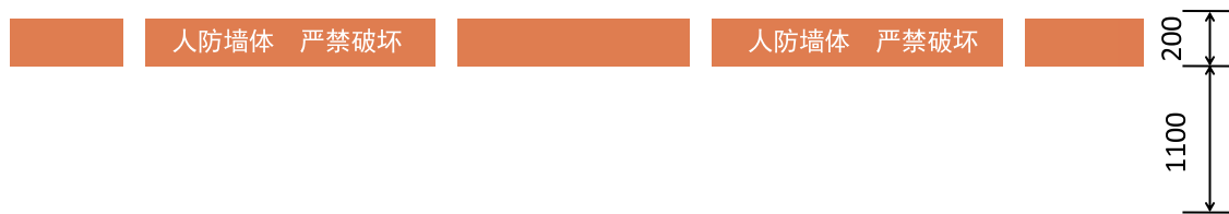
图 21 超配建区墙体标识样式及尺寸示例
