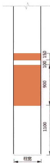
图 22 超配建区柱体标识样式及尺寸示例
